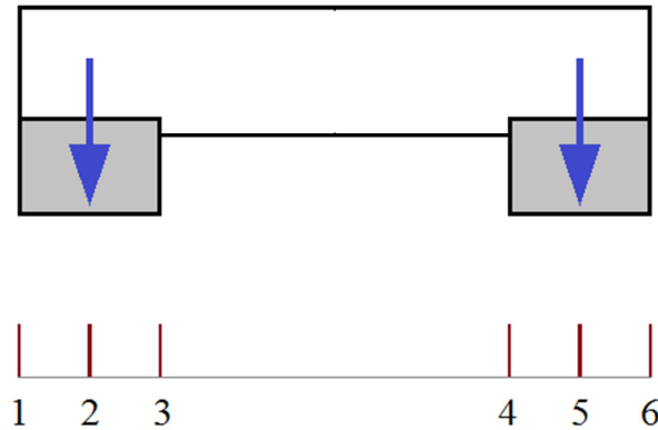
Рис. 14.11. Используемые линии влияния для прокатки подвижных нагрузок АК и НК
